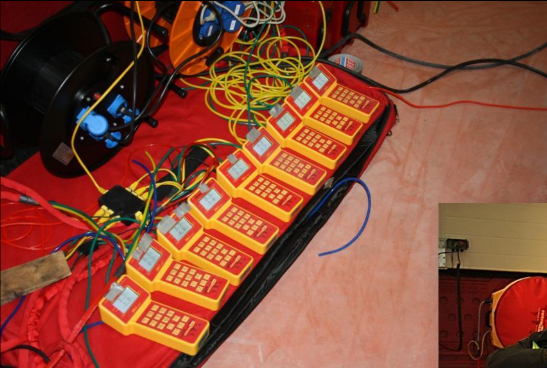
9 x 2-Kanaldruckmessdosen mit Referenzschlauch ins Gebäudeinnere
